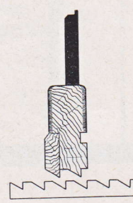
OUTIL POUR FAIRE DES CRÉMAILLÈRES
